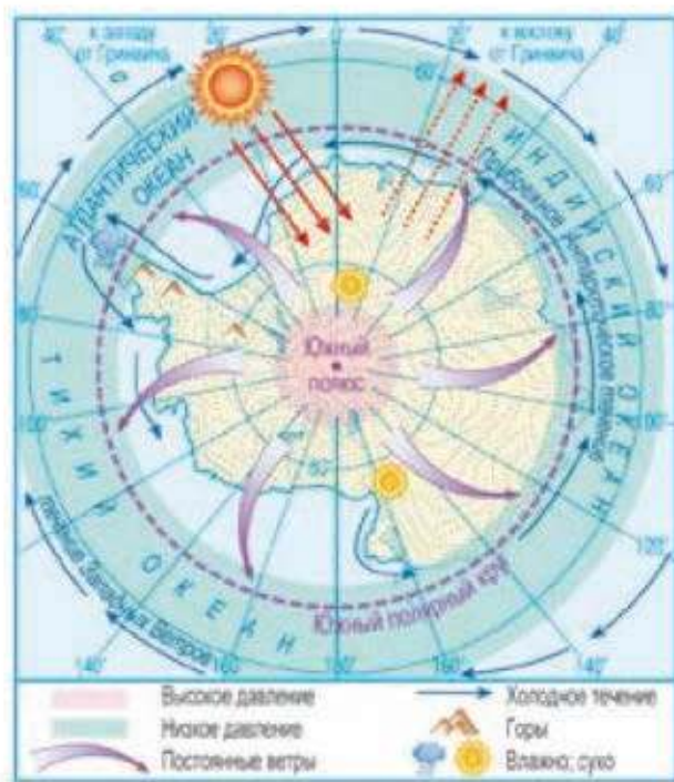
Рис. 100. Климатообразующие факторы Антарктиды
