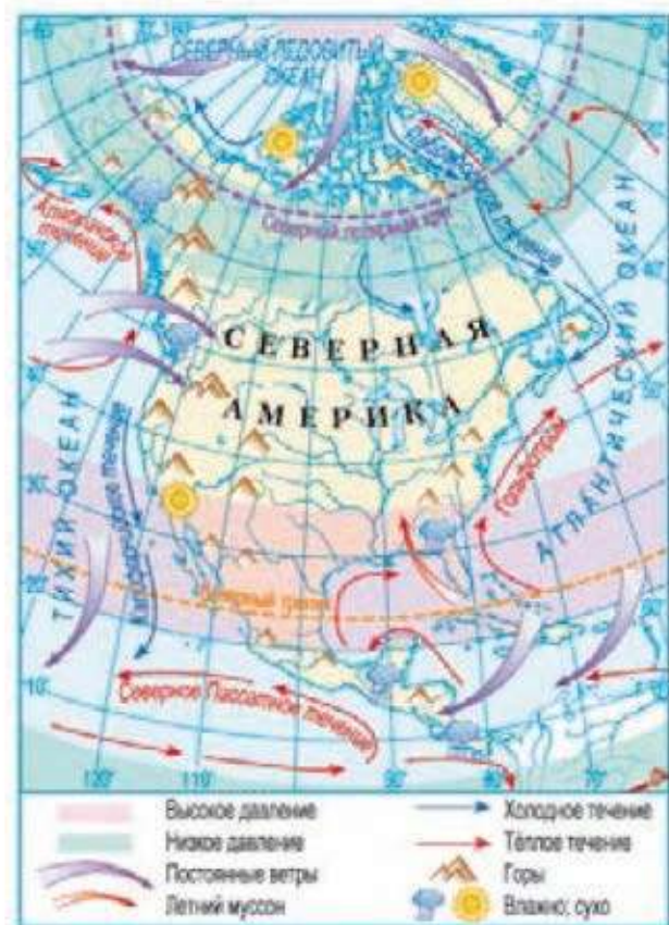
Рис. 152. Климатообразующие факторы Северной Америки
