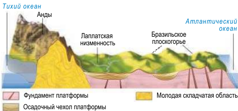
Рис. 112. Строение земной коры и рельеф Южной Америки по 20° ю. ш.
