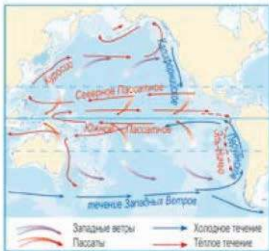
Рис. 42. Круговороты течений в Тихом океане
