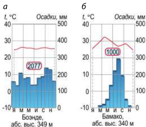
Рис. 58. Климатограммы Африки: а — экваториального, б — субэкваториального муссонного типов климата
