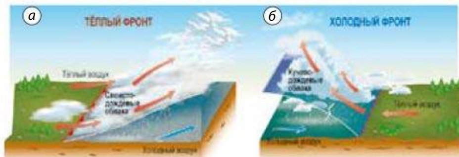
Рис. 15. Образование фронтов: а — тёплого, б — холодного
