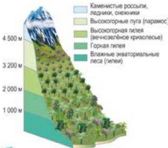
Рис. 137. Высотная поясность Анд в экваториальных широтах
