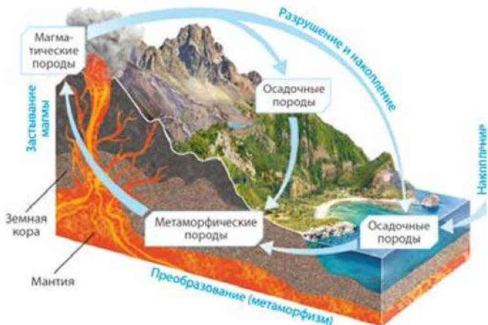
Рис. 2. Геологический круговорот Правообладатель Адукаця і выхаванне
