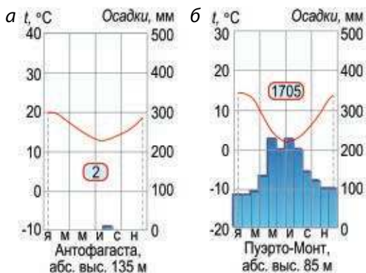
Рис. 122. Климатограммы Южной Америки: а — гаруа, б — умеренного морского типа климата
