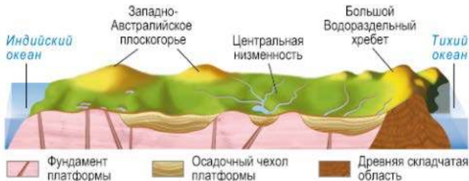
Рис. 78. Строение земной коры и рельеф Австралии по 30° ю. ш.
