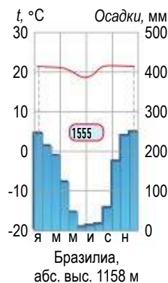
Рис. 19. Климатограмма субэкваториального типа климата
