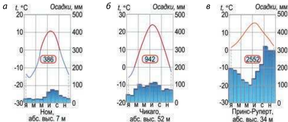
Рис. 153. Климатограммы Северной Америки: а — субарктического морского, б — умеренного континентального, в — умеренного морского типов климата
