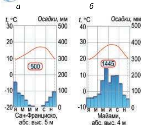
Рис. 155. Климатограммы Северной Америки: а — средиземноморского, б — тропического влажного типов климата
