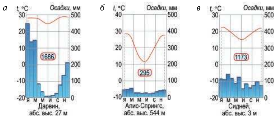
Рис. 87. Климатограммы Австралии: а — субэкваториального муссонного, б — тропического пустынного, в — субтропического влажного типов климата
