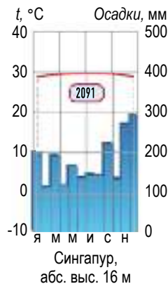
Рис. 18. Климатограмма экваториального типа климата
