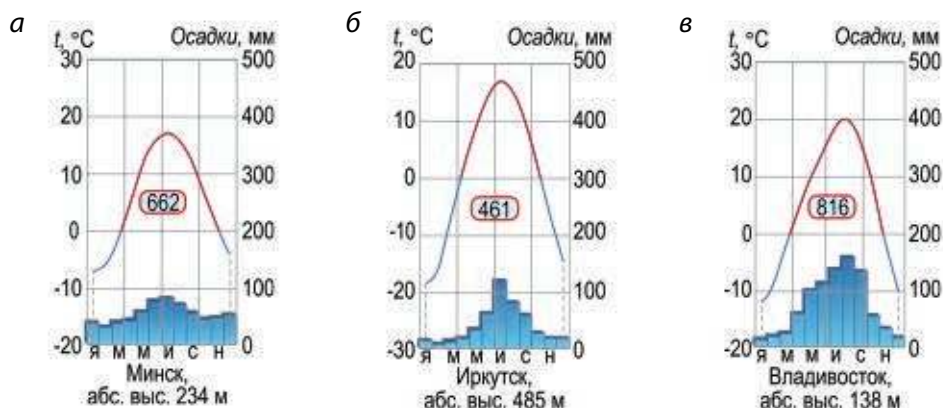
Рис. 192. Климатограммы Евразии: а — умеренно континентального, б — резко континентального, в — умеренного муссонного типов климата
