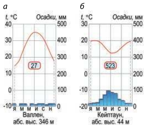
Рис. 60. Климатограммы Африки: а — тропического пустынного, б — средиземноморского типов климата
