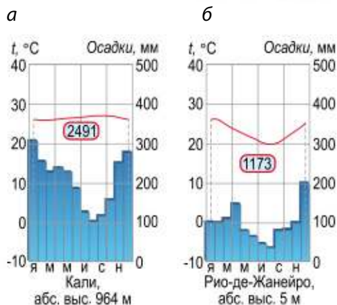
Рис. 121. Климатограммы Южной Америки: а — экваториального, б — тропического влажного типов климата
