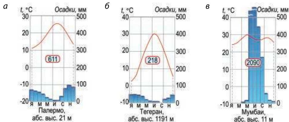
Рис. 193. Климатограммы Евразии: а — средиземноморского, б — субтропического континентального, в — субэкваториального муссонного типов климата
