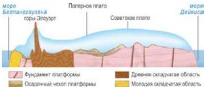
Рис. 98. Строение земной коры и рельеф Антарктиды по 88° з. д. и 92° в. д.
