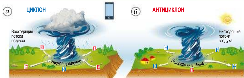
Рис. 16. Формирование циклона (а) и антициклона (б) в Северном полушарии
