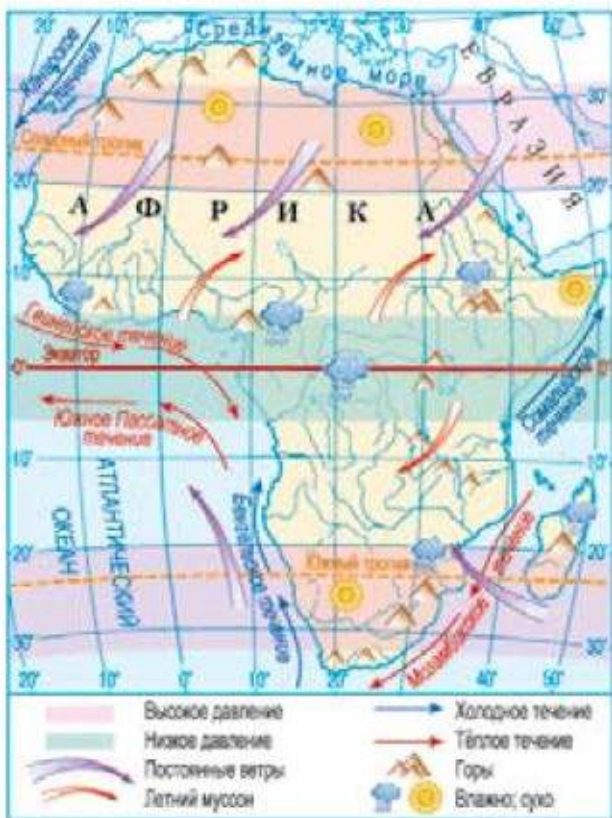
Рис. 57. Климатообразующие факторы Африки
