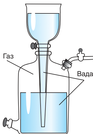
Мал. 6. Газаметр
