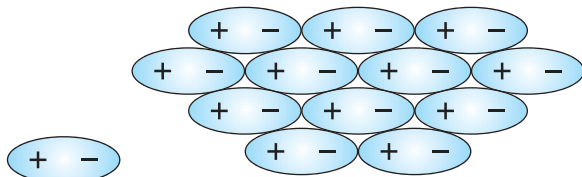
Мал. 74. Дыполь і ўзаемадзеянне дыполяў
