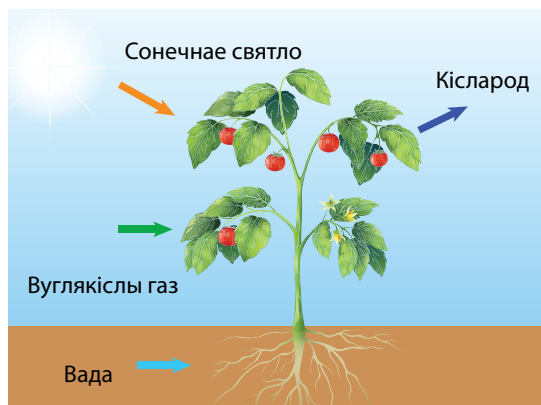
Мал. 86. Утварэнне кіслароду ў выніку фотасінтэзу
