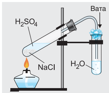
Мал. 28. Атрыманне хлоравадароднай (саянай) кіслаты
