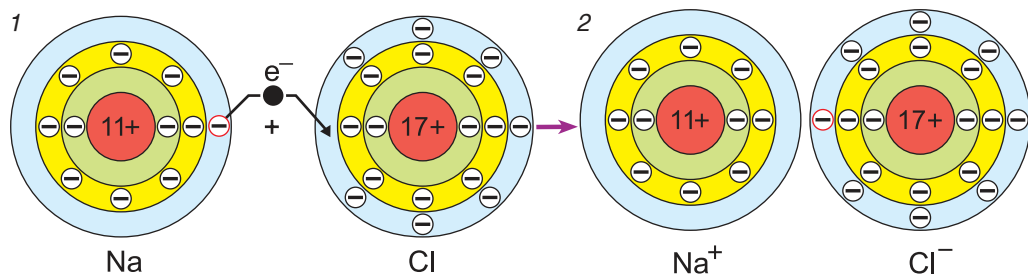
Мал. 70. Схема ўзаемадзеяння атамаў натрыю і хлору: 1 — зыходны стан атамаў, 2 — электронная будова іонаў Na + і Cl -
