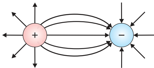
Мал. 71. Сілавая лінія палёў іонаў у іонным крышталі
