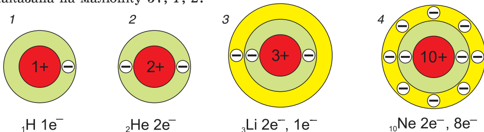
Мал. 57. Электронныя схемы атамаў: 1 — вадароду, 2 — гелію, 3 — літыю, 4 — неону
