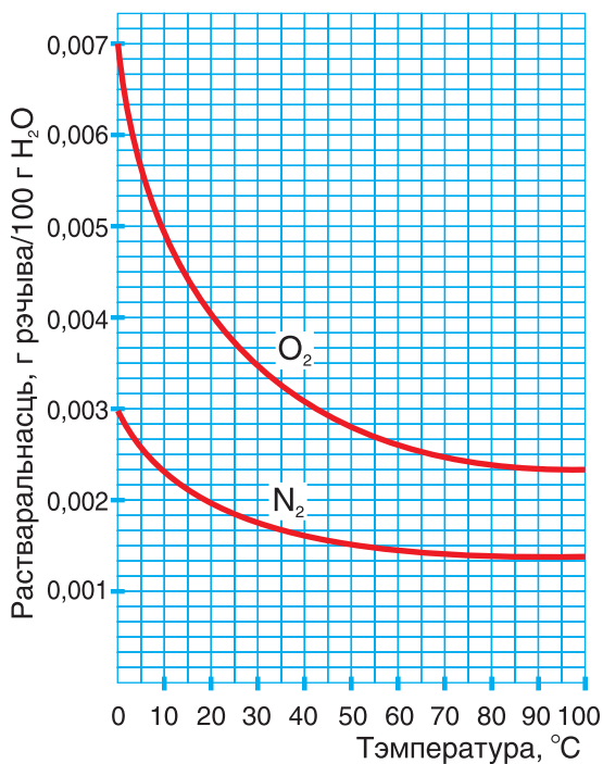
Мал. 108. Залежнасць растваральнасці газаў — кіслароду і азоту ад тэмпературы
