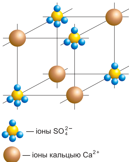
Мал. 78. Фрагмент крышталічнай рашоткі сульфату кальцыю \text{CaSO}_4
