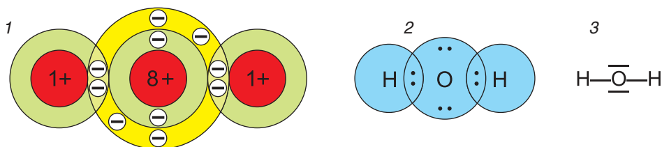
Мал. 99. Электронная будова малекулы вады: 1 — утварэнне кавалентных сувязей, 2 — электронная формула, 3 — графічная формула
