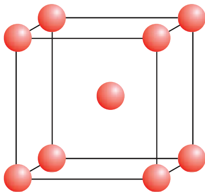
Мал. 79. Фрагмент крышталічнай рашоткі натрыю Na
