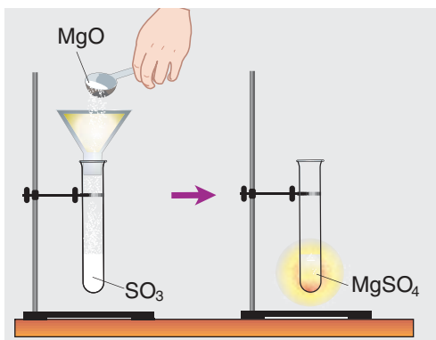
Мал. 19. Рэакцыя аксиду магнію з аксідам серы(VI)
