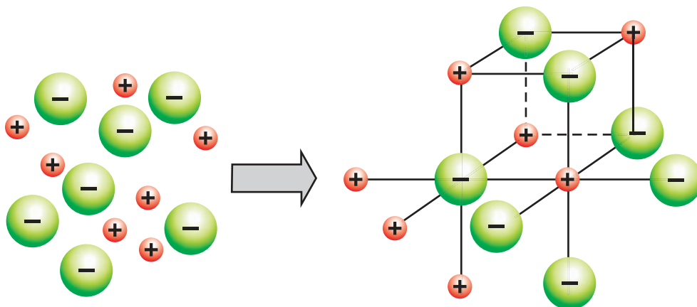
Мал. 75. Утварэнне іоннай крышталічнай структуры хларыду натрыю \text{NaCl}
