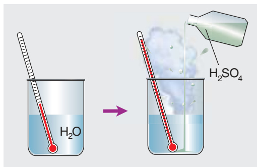
Мал. 104. Павышэнне тэмпературы пры растварэнні ў вадзе сернай кіслаты
