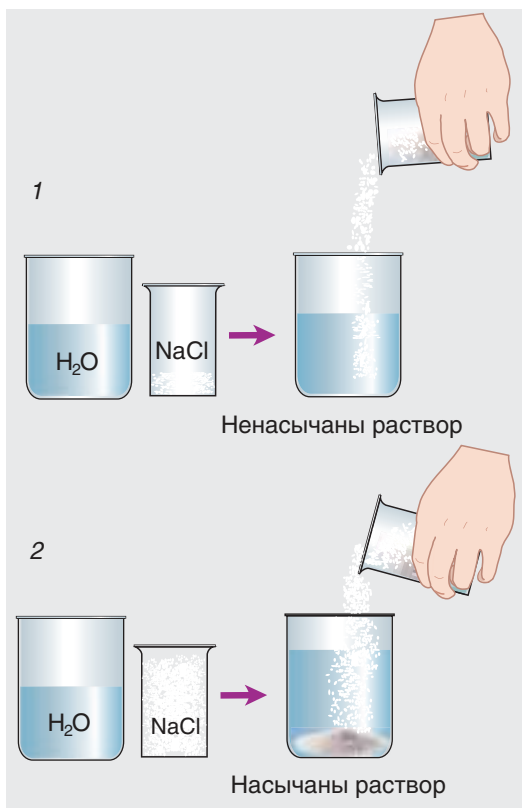
Мал. 111. Ненасычаны (1) і насычаны (2) растворы кухоннай солі
