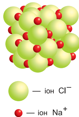
Мал. 72. Іонны крышталёвы хларыд натрыю
