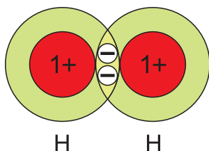
Мал. 64. Схема ўтварэння агульнай электроннай пары ў малекуле вадароду
