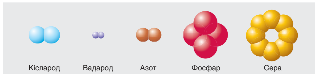
Мал. 1. Шаравыя мадэлі малекул
