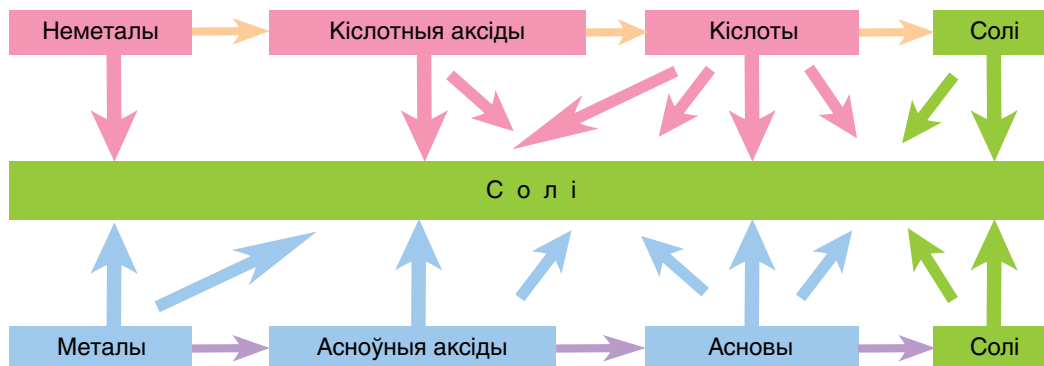
Мал. 38. Схема ператварэнняў неарганічных рэчываў
