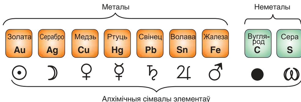
Мал. 39. Хімічныя элементы старажытнасці
