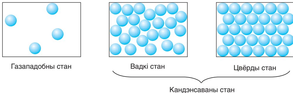
Мал. 10. Схема газападобнага і кандэнсаванага стану рэчываў
