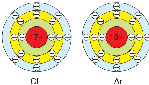
Мал. 66. Схема электроннай будовы атамаў хлору і аргону
