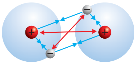
Мал. 61. Схема дзеяння кулонаўскіх сіл у малекуле вадароду \text{H}_2
