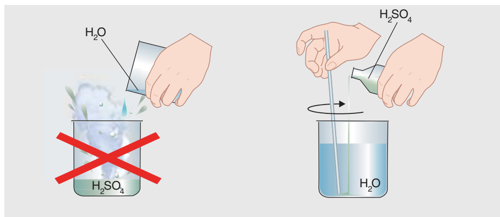
Мал. 30. Падрыхтоўка воднага раствору сернай кіслаты
