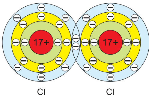
Мал. 67. Схема ўтварэння агульнай электроннай пары ў малекуле хлору
