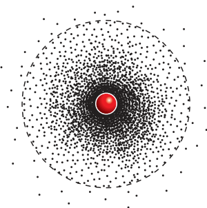
Мал. 54. Электроннае воблака
