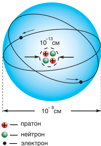
Мал. 50. Мадэль атама гелію
