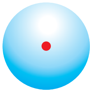
Мал. 55. Арбіталь электрона ў атаме вадароду
