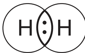
Мал. 65. Электронная формула малекулы вадароду
