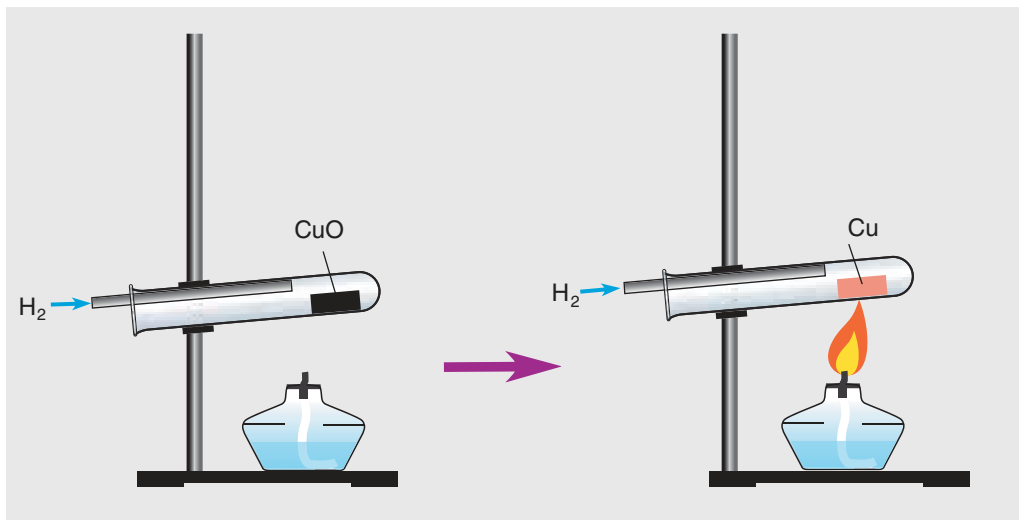
Мал. 83. Утварэнне медзі з аксиду медзі(II)
