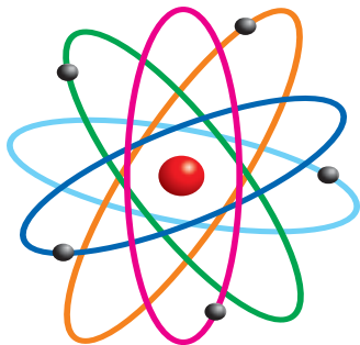
Мал. 49. Ядзерная мадэль атама паводле Рэзерфарда
