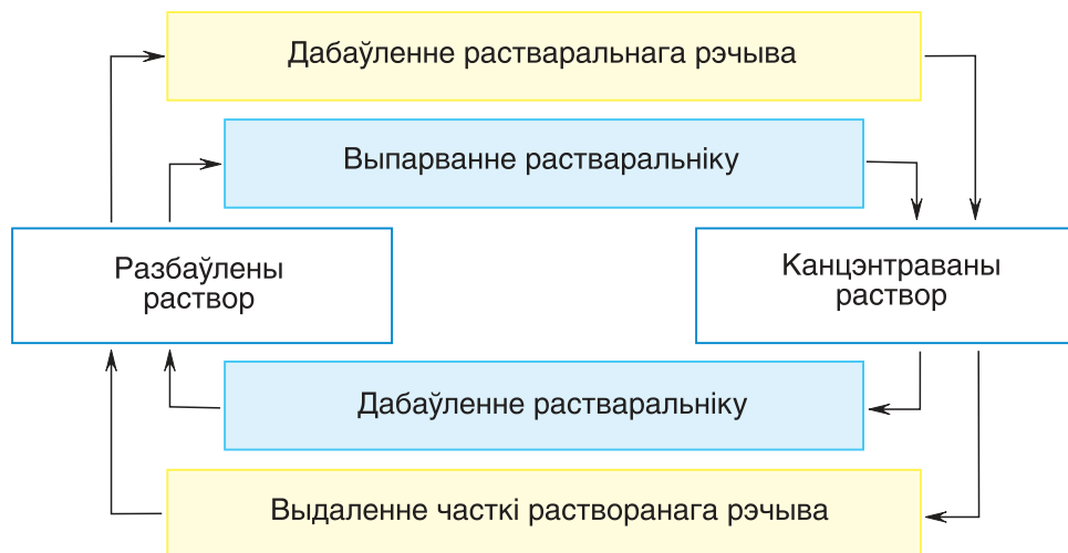
Мал. 113. Спосабы змянення наяўнасці растваранага рэчыва ў растворы
