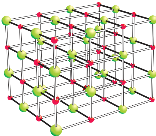
Мал. 76. Фрагмент крышталічнай рашоткі хларыду натрыю \text{NaCl}
