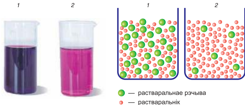
Мал. 112. Канцэнтраваны (1) і разбаўлены (2) растворы перманганату калію і іх мадэлі
