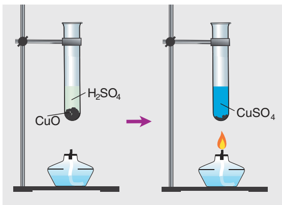
Мал. 25. Рэакцыя сернай кіслаты з аксідам медзі(II)
