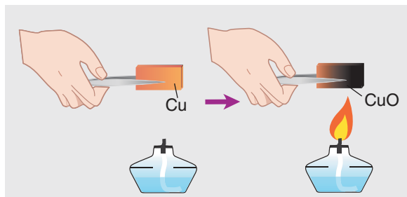
Мал. 82. Утварэнне аксіды медзі на меднай пласцінцы
