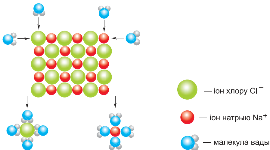
Мал. 105. Утварэнне сувязей паміж часціцамі растваранага рэчыва \text{NaCl} і малекуламі вады \text{H}_2\text{O}
