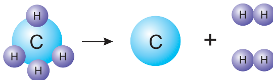
Мал. 14. Схема рэакцыі раскладання
