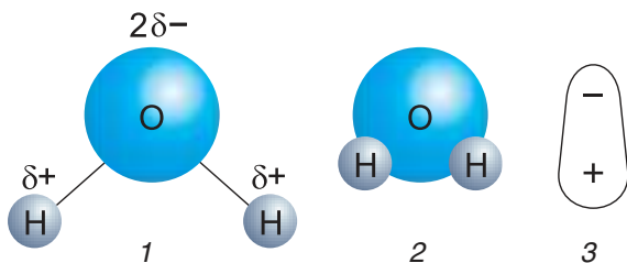
Мал. 100. Молекула вады: 1 — вуглавая структура, 2 — шаравая мадэль, 3 — дыполь
