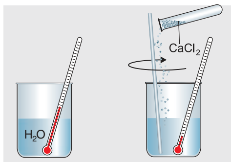
Мал. 103. Паніжэнне тэмпературы пры растварэнні ў вадзе хларыду кальцыю
