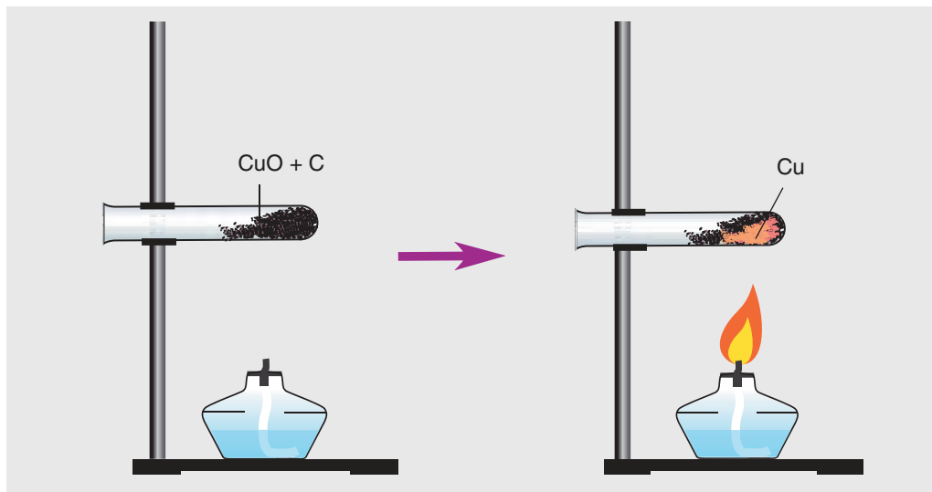
Мал. 89. Аднаўленне медзі з яе аксiду вугляродам
