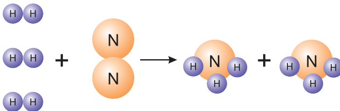
Мал. 15. Схема рэакцыі злучэння
