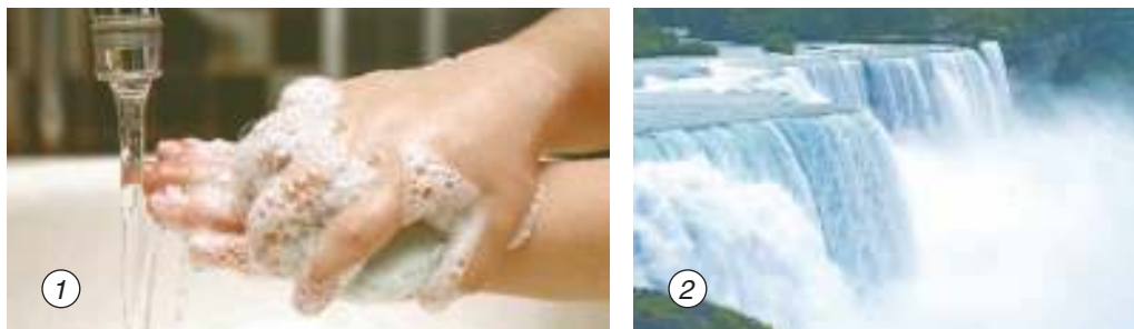
Мал. 94. Пена — завісць газу ў вадкасці: 1 — мыльная пена, 2 — вадаспад
