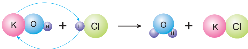
Мал. 17. Схема рэакцыі абмену
