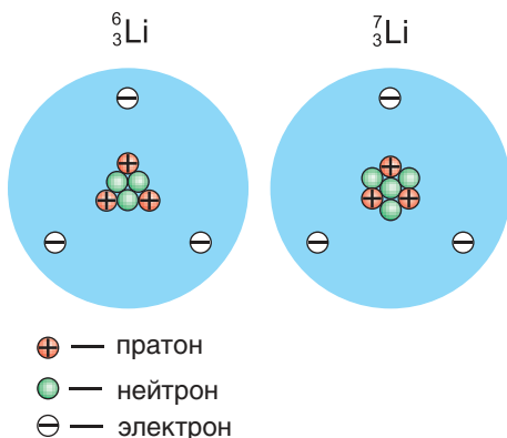
Мал. 51. Мадэлі нуклідаў літыю
