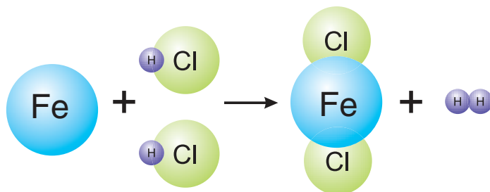
Мал. 16. Схема рэакцыі замяшчэння
