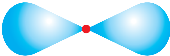
Мал. 56. Форма адной з арбіталей у шматэлектронным атаме
