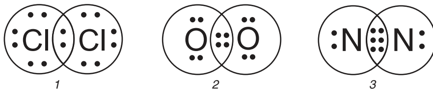
Мал. 68. Электронныя формулы малекул: 1 — хлору, 2 — кіслароду, 3 — азоту
