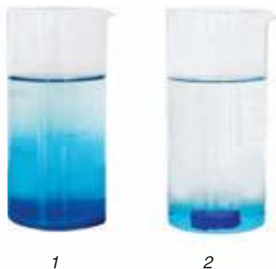
Мал. 109. Растварэнне ў вадзе парашку (1) і крышталёў (2) меднага купарвасу аднолькавай масы
