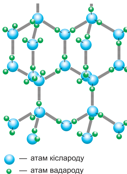
Мал. 81. Фрагмент крышталічнай рашоткі лёду H_2O
