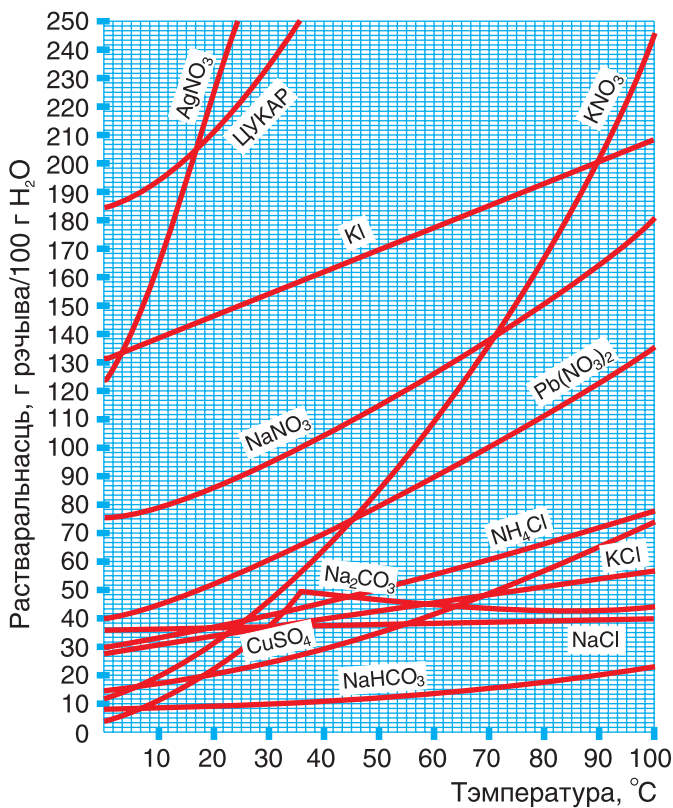
Мал. 107. Залежнасць растваральнасці некаторых цвёрдых рэчываў ад тэмпературы
