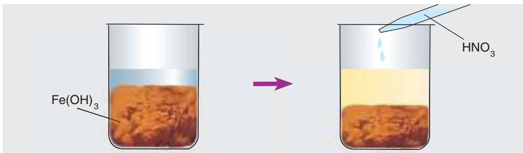
Мал. 26. Рэакцыя азотнай кіслаты з гідраксідам жалеза(III)
