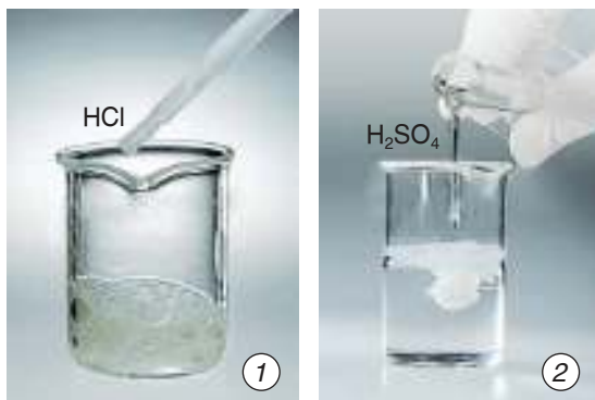
Мал. 27. Рэакцыі: 1 — сялянай кіслаты з сульфідам калію, 2 — сернай кіслаты з хларыдам барыю
