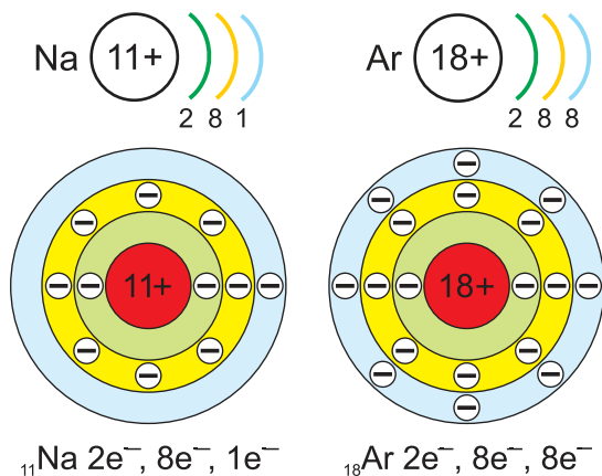
Мал. 58. Электронныя схемы атамаў натрыю і аргону (уверсе — спрошчаны выгляд схем)
