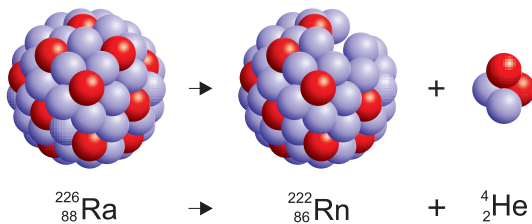
Мал. 52. Схема распаду ядра атама радыю
