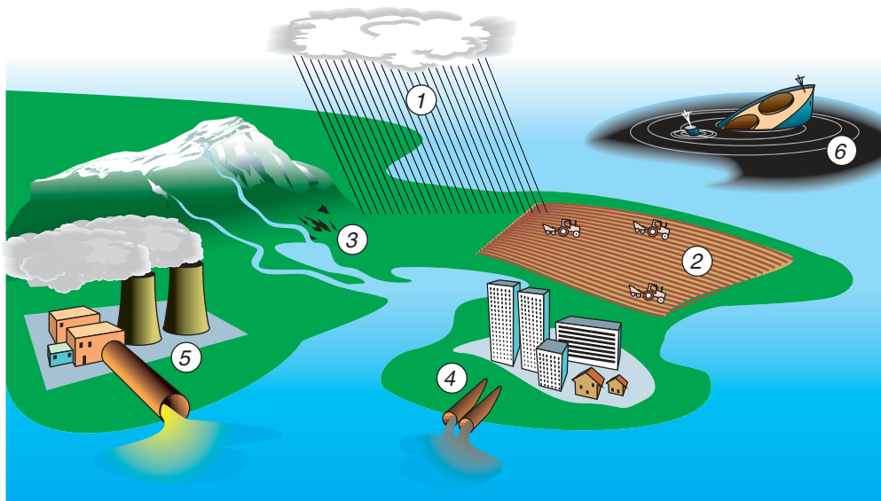
Мал. 119. Асноўныя крыніцы забруджвання вады: 1 — кіслотныя дажджы, 2 — мінеральныя ўгнаенні і сродкі аховы раслін, 3 — адвалы горных парод і адходаў вытворчасцей, звалкі смецця, 4 — бытавыя сцёкі, 5 — прамысловыя адходы, 6 — катастрофы нафтаналіўных суднаў
