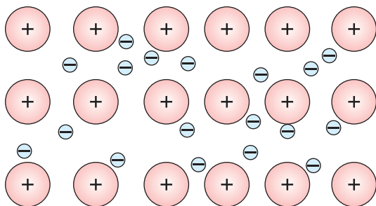
Мал. 73. Схема будовы крышталю металу
