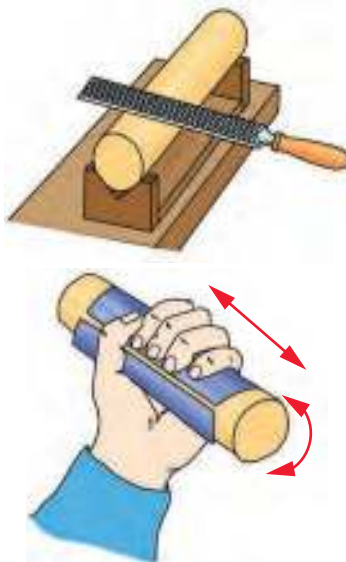
Рис. 33. Шлифование детали цилиндрической формы
