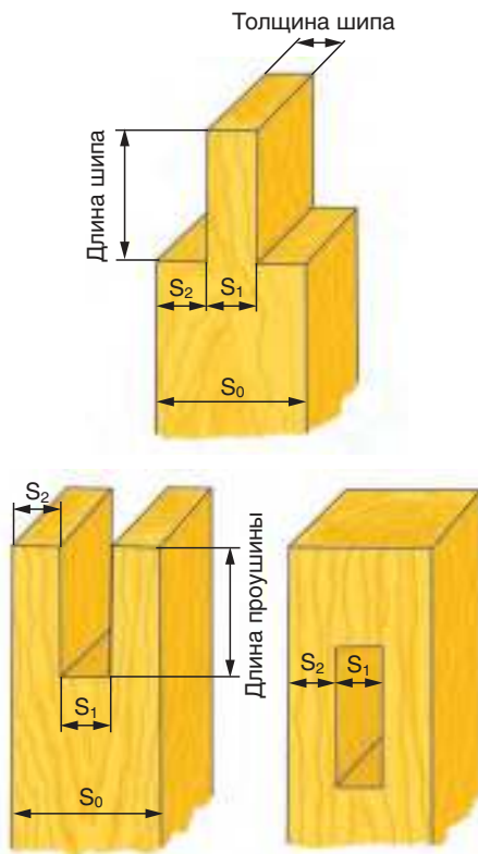
Рис. 11. Параметры шипового соединения
