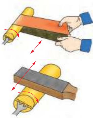
Рис. 47. Шлифование поверхности: шлифовальной шкуркой (вверху) и бруском со шлифовальной шкуркой (внизу)
