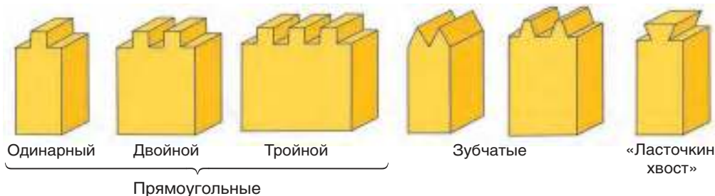
Рис. 10. Виды шипов
