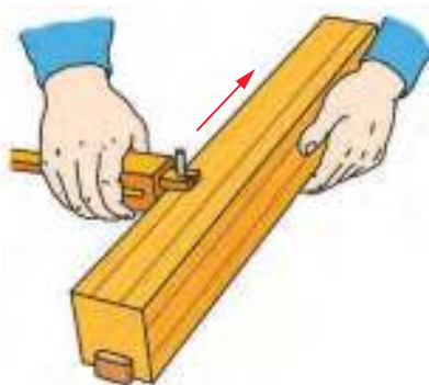
Разметка рейсмусом
