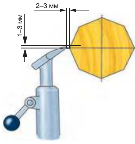
Рис. 42. Установка подручника
