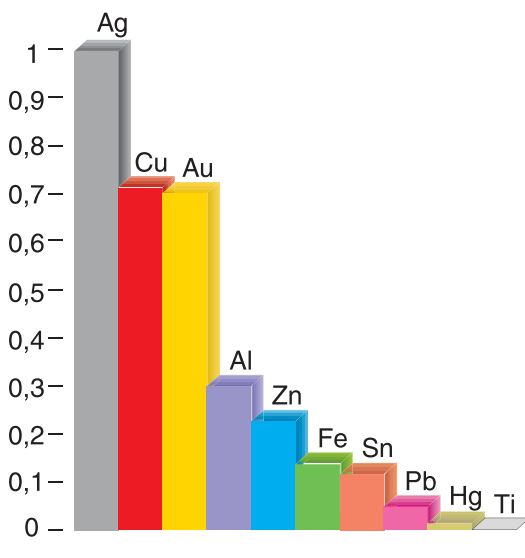
Рис. 120. Сравнительная электропроводность металлов
