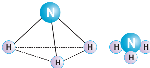
Рис. 68. Модель молекулы аммиака
