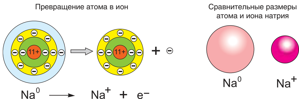
Рис. 19. Схема электронного строения атома и иона натрия
