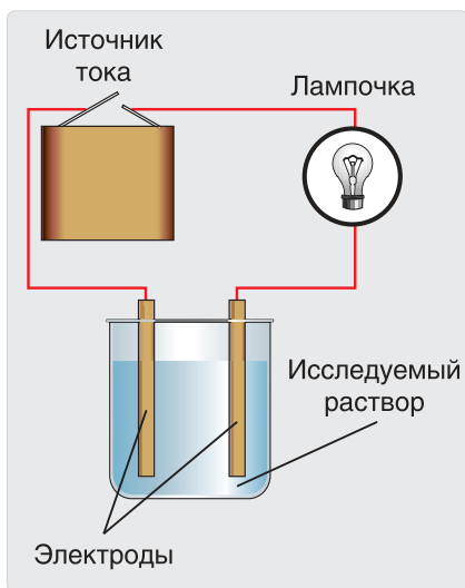
Рис. 14. Схема прибора для определения электропроводности раствора
