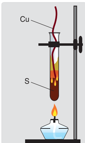
Рис. 55. Взаимодействие серы с медью
