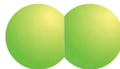
Рис. 35. Модель молекулы хлора
