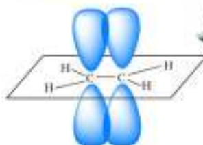
этилен
