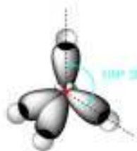
метан
