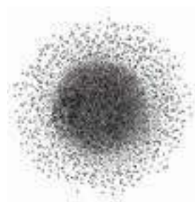
Рис. 1.4. Электронное облако атома водорода
