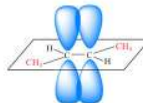
транс-бутен-2
