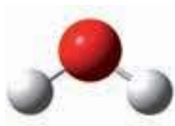
Рис. 1.1. Модель молекулы воды
