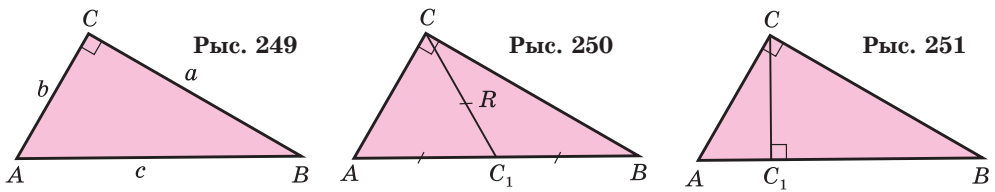
Прамавугольны трохвугольнік (гл. рыс. 249) мае такія ўласцівасці:
