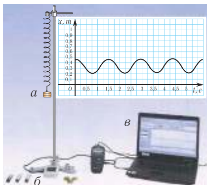
Мал. 6. Устаноўка для запісу асцылаграмы ваганняў маятніка: а — груз на sprужыне; б — ультрагукавы датчык руху; в — ноутбук
