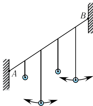
Мал. 27. Назіранне з'явы рэзанансу ў сістэме маятнікаў
