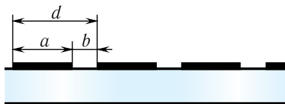
Мал. 96. Дыфракцыйная рашотка
