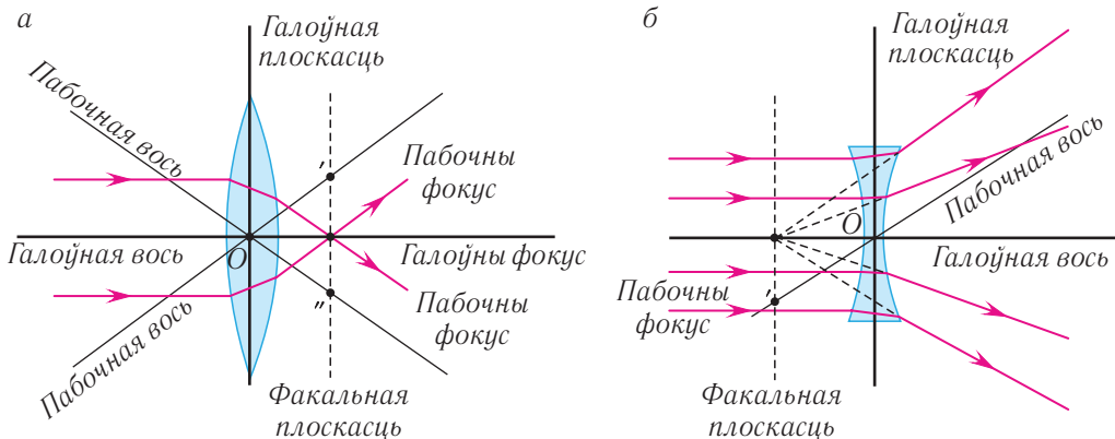
Мал. 148. Асноўныя характарыстыкі лінзы:
