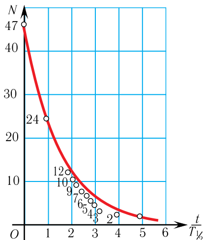
Мал. 219. Лік ядзер ^{256}_{100}\text{Fm} , што не распаліся, у залежнасці ад часу
