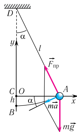
Мал. 16. Сілы, што дзейнічаюць на матэматычны маятнік
