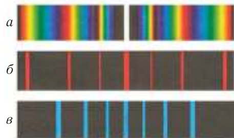
Мал. 99. а — дыфракцыйны спектр белага святла; б — дыфракцыйныя максімуі чырвонага святла; в — дыфракцыйныя максімуі сіняга святла
