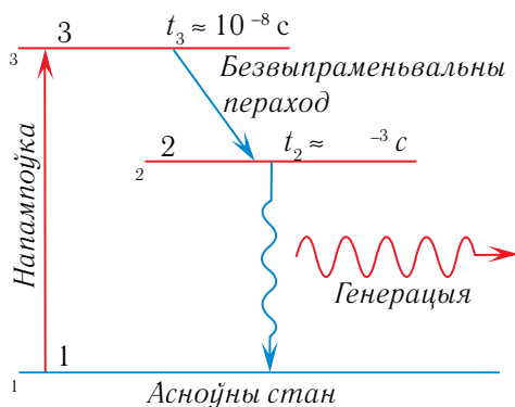
Мал. 205. Трэхузроўневая схема генерацыі вымушанага выпраменьвання
