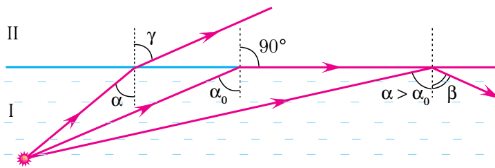
Мал. 132. Прамаленне і адбіццё святла на мяжы падзелу асяроддзяў
