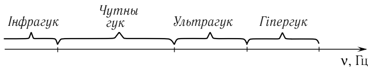
Мал. 41. Шкала гукавых хваль
