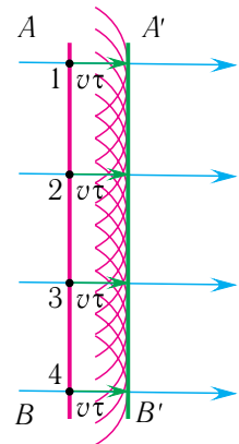
Мал. 94. Прамалінейнае распаўсюджванне хваль (фарміраванне фронту плоскай хвалі)
