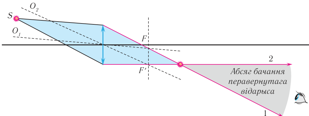
Мал. 151. Пабудова відарыса ў збіральнай лінзе і абсяг бачання
