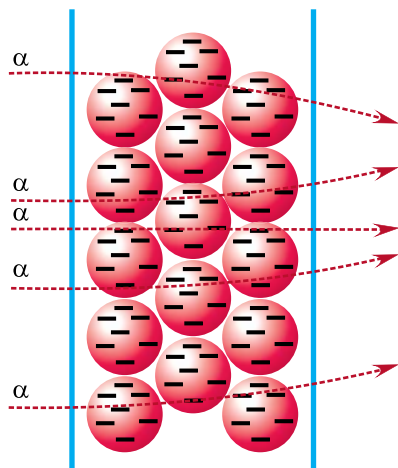
Мал. 188. Меркаванае рассяйванне \alpha -часціц атамамі золата паводле мадэлі Томсана
