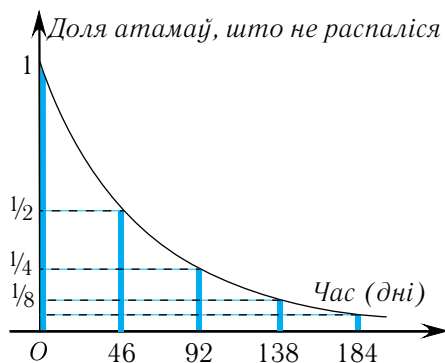
Мал. 218. Радыеактыўны распад нукліда жалеза ^{59}_{28}\text{Fe}
