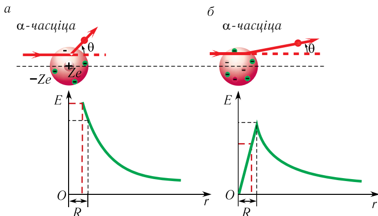
Мал. 190. Мадэлі атама і залежнасці модуля напружанасці электрычнага поля ад адлегласці: а — ядзерная мадэль; б — мадэль атама Томсана
