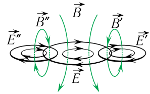
Мал. 73. Утварэнне електрамагнітнай хвалі
