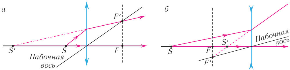
Мал. 150. Пабудова відарыса з дапамогай пабочнай аптычнай восі: a — збіральная лінза; b — расейвальная лінза
