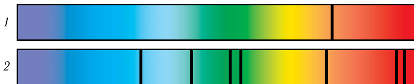
Мал. 202. Спектры паглынання розных рэчываў: 1 — натрыю; 2 — гелію
