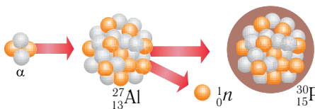
Мал. 215. Ператварэнне алюмінію ў радыеактыўны ізотоп фосфару
