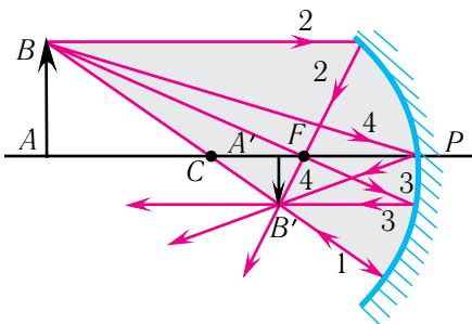
Мал. 116. Стандартныя промяні ў сфэрычным люстры
