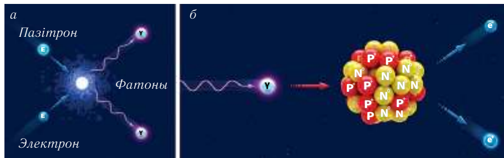
Мал. 231. а — анігіляцыя электрона і пазітрона пры сутыкненні; б — нараджэнне электронна-позітроннай пары з \gamma -кванта ў полі ядра
