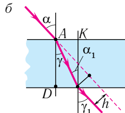
Мал. 138. а — светлавы прамень, які праходзіць праз плоскапаралельную пласцінку; б — ход праменя ў пласцінцы
