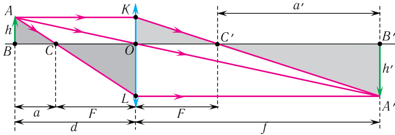
Мал. 153. Да виваду формулы лінзы
