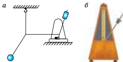
Мал. 25. a — назіранне з'явы рэзанансу ў сістэме матэматычны маятнік — метраном; б — знешні выгляд метранома
