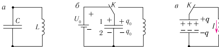
Мал. 52. а — вагальны контур; б — зарадка кандэнсатара ад крыніцы; в — праходжанне току па контуры
