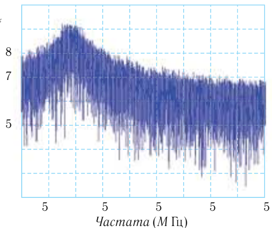
Мал. 45. Спектр шуму
