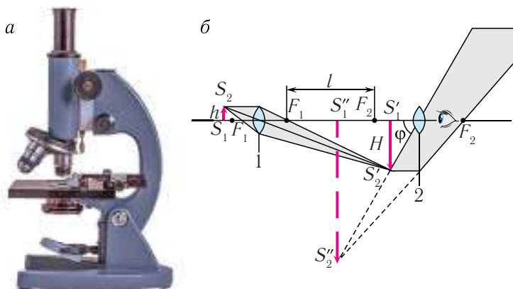
Мал. 163. Мікраскоп: а — агульны выгляд; б — аптычная схема і ход праменяў
