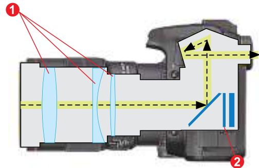
Мал. 158. Лічбавы фотаапарат і яго аптычная схема: 1 — сістэма лінз (аб'ектыў); 2 — святлоадчувальная матрыца
