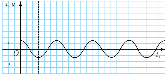
Мал. 7. Асцылаграма ваганняў грузу на sprужыне
