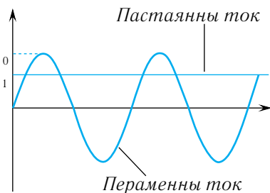
Мал. 60. Графік залежнасці сілы току I ад часу t вагальным контуры і дзеючае значэнне пераменнага току
