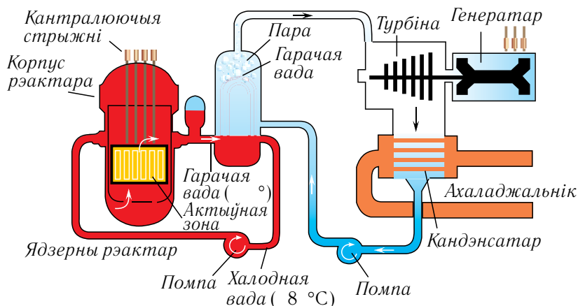
Мал. 226. Дыяграма, якая паказвае работу атамнай электрастанцыі з герметычным вадзяным контурам ахаладжвання
