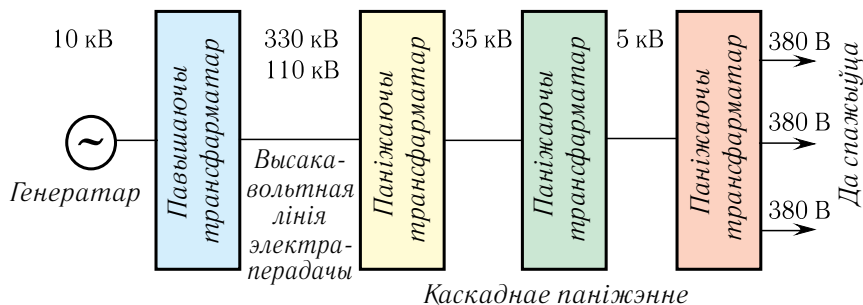
Мал. 69. Блок-схема перадачы электраэнергіі
