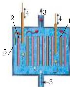
Мал. 225. Схема актыўнай зоны рэактара: 1 — актыўная зона з цвяламі; 2 — запавольнік (вада); 3 — сістэма адводу цепланосьбіта; 4 — стрыжні кіравання рэакцыяй; 5 — ахоўны корпус
