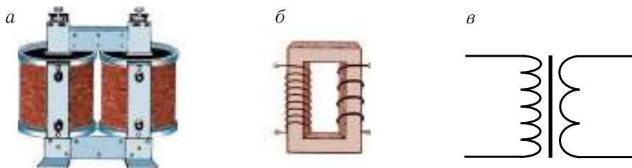
Мал. 65. Трансфарматар:
