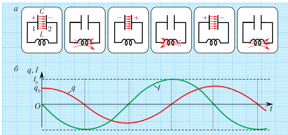
Мал. 53. a — электрамагнітныя ваганні ў ідэальным LC -контуры; б — залежнасці зараду кандэнсатара q , сілы току I ў шпулі ад часу
