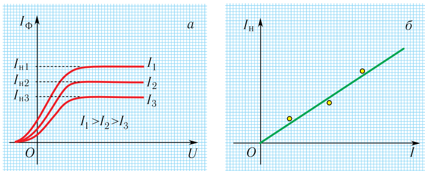
Мал. 173. а — вольт-амперная характарыстыка фотаэфекту пры розных інтэнсіўнасцях падаючага выпраменьвання; б — залежнасць сілы фотатоку насычэння ад інтэнсіўнасці падаючага выпраменьвання
