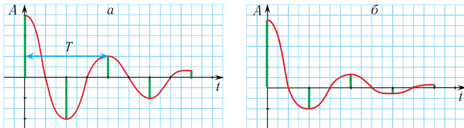
Мал. 24. Затухаючыя механічныя ваганні (каэфіцыенты трэння (супраціўлення) \mu_a < \mu_6 ): a — малая сіла трэння; б — вялікая сіла трэння
