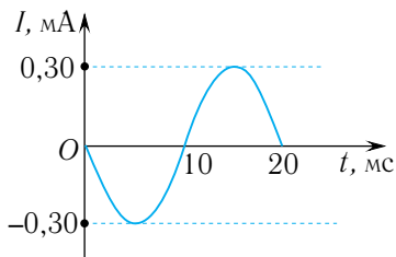
Мал. 62. Графік залежнасці сілы току I ад часу ў вадзільным контуры
