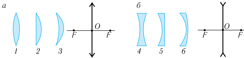
Мал. 147. Типы линз і їх умовні абазначэнні: а — збіральныя:
