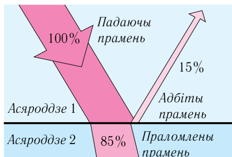
Мал. 131. Баланс энергій пры адбіцці і праламненні святла на мяжы падзелу празрыстых асяроддзяў
