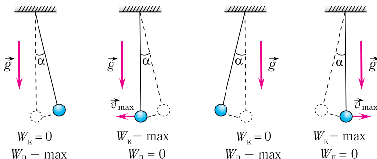
Мал. 19. Пераўтварэнні энергіі пры ваганнях матэматычнага маятніка
