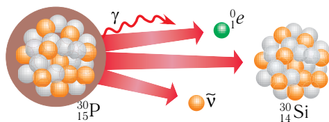
Мал. 216. Распад радыеактыўнага ізатопа фосфару з утварэннем крэмнію і выпусканнем пазітрона
