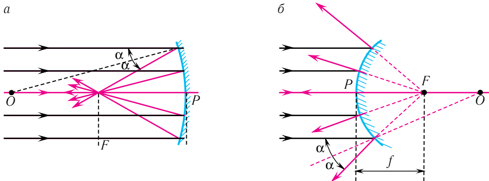
Мал. 114. Побудова ходу променяў, паралельных галоўнай аптычнай восі, у люстрах: а — увагнутым; б — выпуклым
