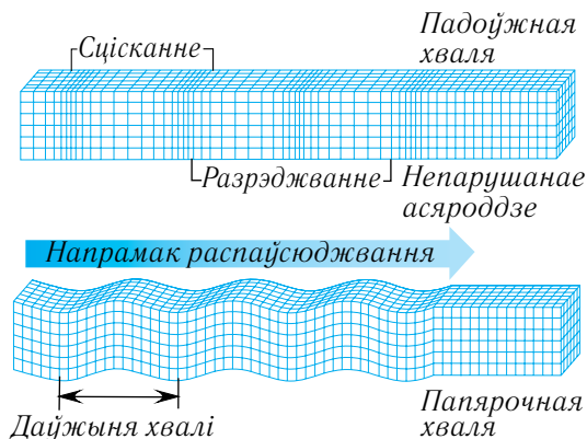
Мал. 39. Падоўжныя і папярочныя хвалі
