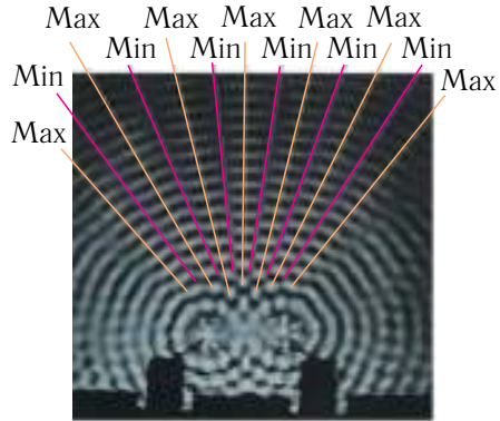
Мал. 88. Інтэрферэнцыйная карціна папяровых хваль на паверхні вады
