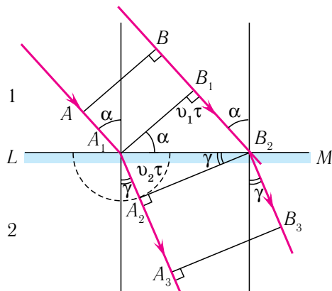
Мал. 130. Тлумачэнне праламлення святла ў адпаведнасці з прынцыпам Гюйгенса: AB — фронт падаючай плоскай хвалі; A_2B_2 — фронт хвалі пасля праламлення
