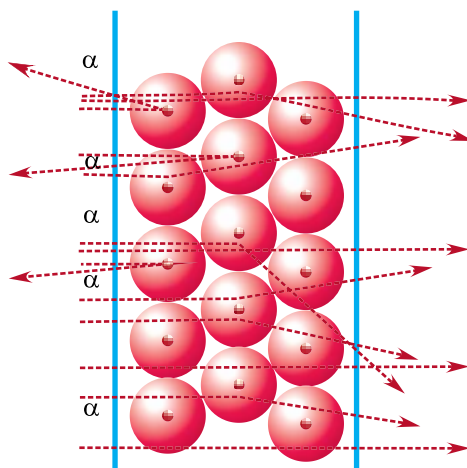
Мал. 189. Назіраемае рассяйванне \alpha -часціц у доследах Рэзерфарда
