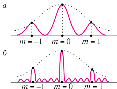
Мал. 100. Змяненне дыфракцыйнай карціны пры павелічэнні колькасці шчылін: а — дзве шчыліны; б — шэсць шчылін
