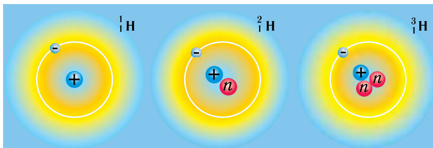
Мал. 210. Тры ізаотопы вадароду
