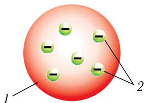
Мал. 186. Мадэль атама Томсана:
