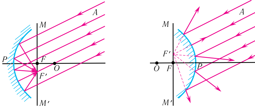
Мал. 115. Адбіццё пучка промяняў, паралельных пабочнай аптычнай восі
