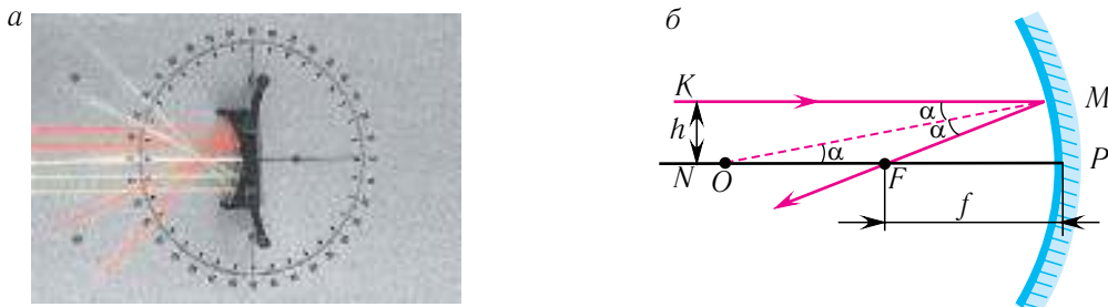
Мал. 113. Увагнутае сферычнае люстра:
