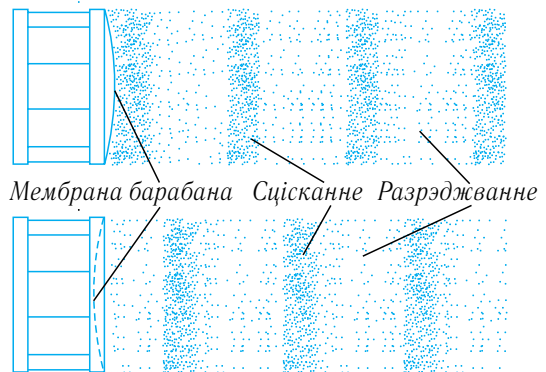
Мал. 42. Утварэнне гукавой хвалі, ствараемай мембранай барабана
