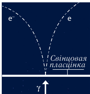
Мал. 232. Нараджэнне электронна-позитроннай пары з \gamma -кванта пры праходжанні квантаў праз свінцовую пласцінку
