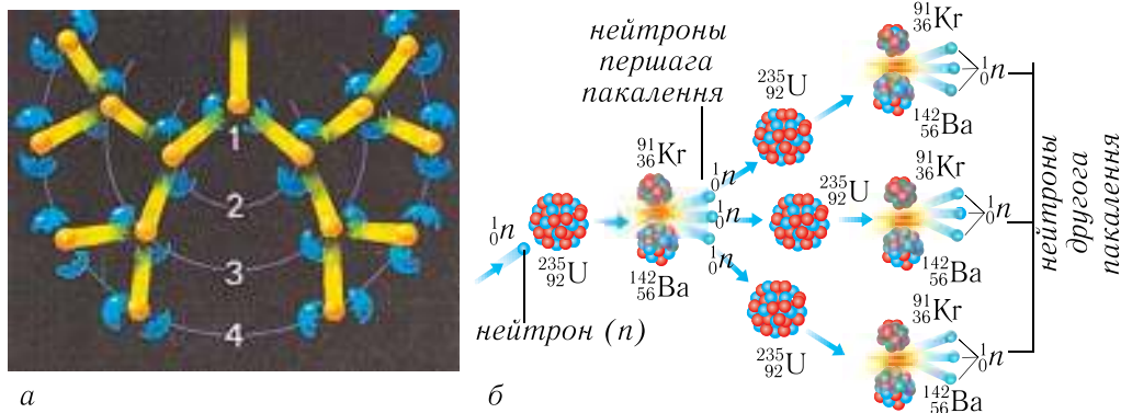
Мал. 221. a — ланцуговая рэакцыя дзялення (1 — першасны нейтрон (першае пакаленне), 2 — другое пакаленне, 3 — трэцяе пакаленне); б — схема рэакцыі
