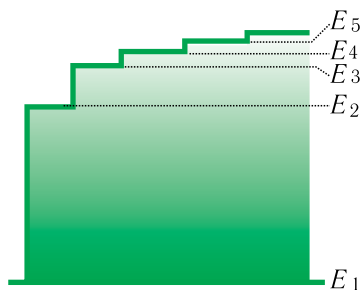
Мал. 196. Энергетычная «лесвіца» станаў атама вадароду
