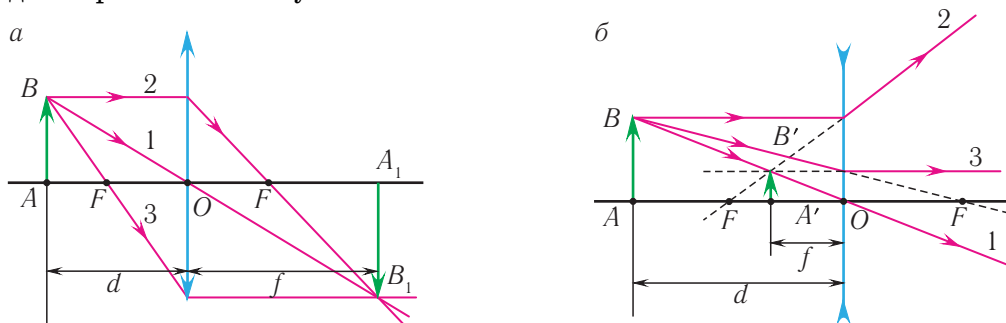
Мал. 149. Стандартныя прамені для пабудовы ў лінзах:
