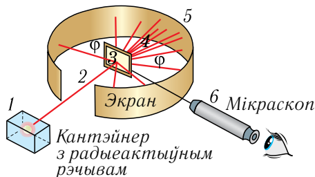
Мал. 187. Схема эксперыментальнай устаноўкі Рэзерфарда па рассеянні \alpha -часціц:
