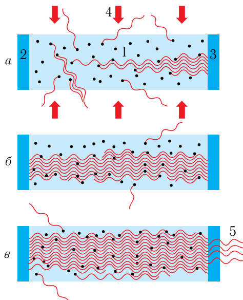
Мал. 206. Прынцыповая схема лазера на рубіне: 1 — актыўнае асяроддзе; 2 — цалкам адбіваючае люстра; 3 — паўпразрачнае люстра; 4 — напампоўка; 5 — генерыруемае выпраменьванне
