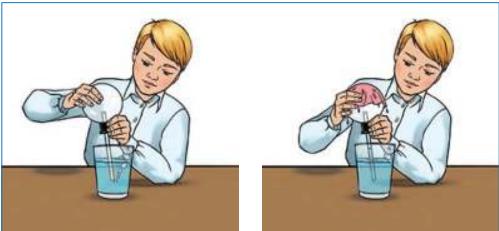
Мал. 70. Вопыт, які даказвае, што паветра пры награванні пашыраецца, а пры ахаладжэнні сціскаецца
