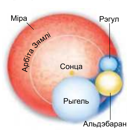
Мал. 12. Параўнальныя памеры зорак
